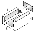
5504/5506 Stopp ende. Sett med to stk. 244x300x200 | 140
