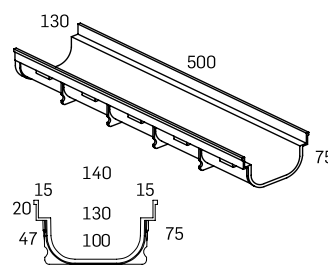
C075 130G Renne for lukket kanalsystem 500 x 130 x 75 mm
