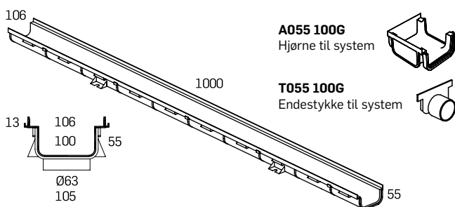
C055 100G Renne for lukket kanalsystem 1000 x 106 x 55 mm
